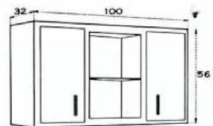
Type PIW
